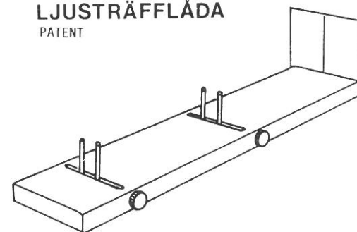
MÄTJIGG
